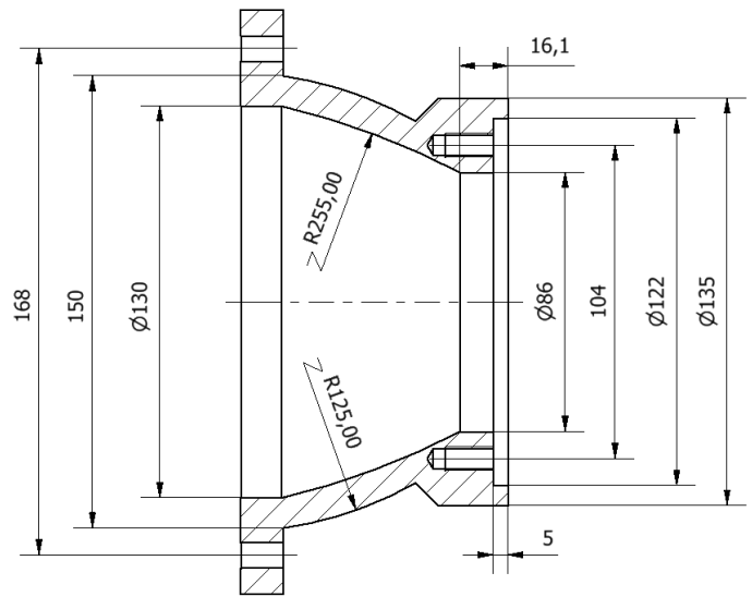
A-A (1:2)
