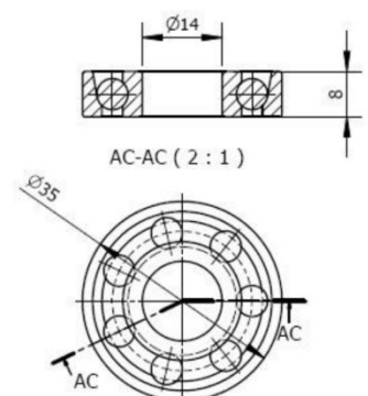
BALL BEARING JIS B 1538 EN 14 14x35x8
